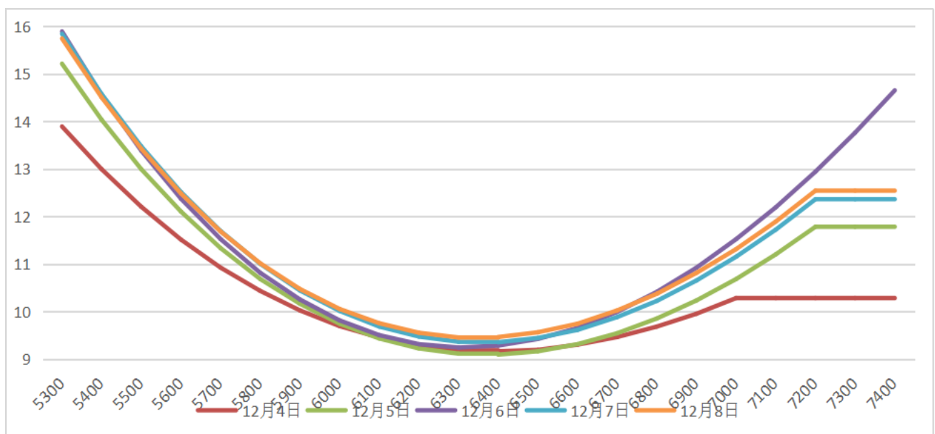
图3 白糖805合约隐含波动率分布图
